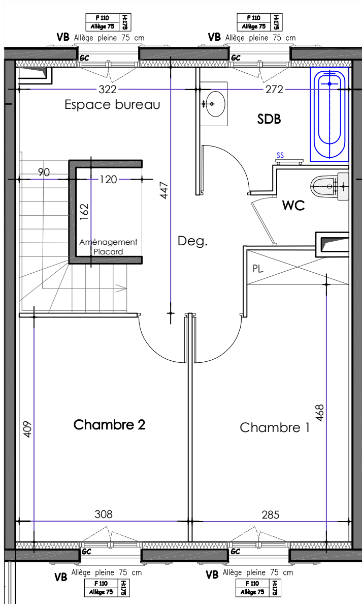
Plan 2ème Etage
